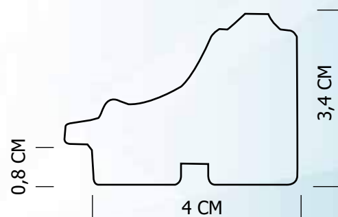
SEZIONE CORNICE SCALA 1:1
