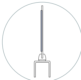
DETTAGLIO PROFILO
